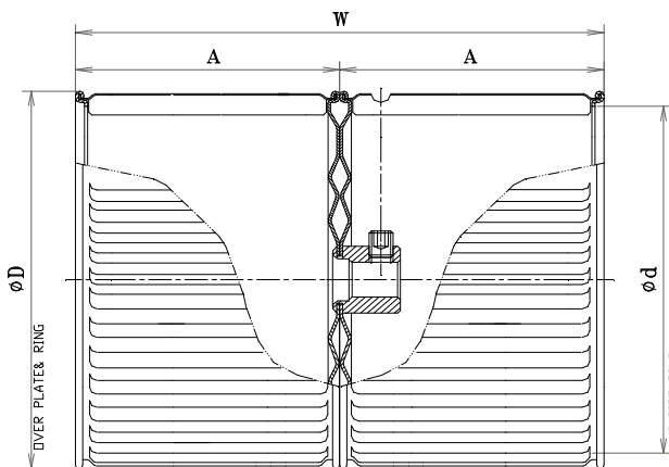
TYPE : N Double Inlet
