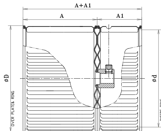
TYPE : N Double Inlet
